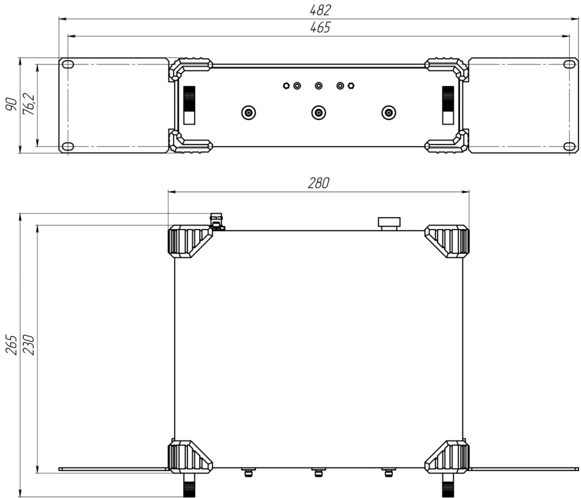
Рис.3. Чертёж. (Все размеры в миллиметрах).
